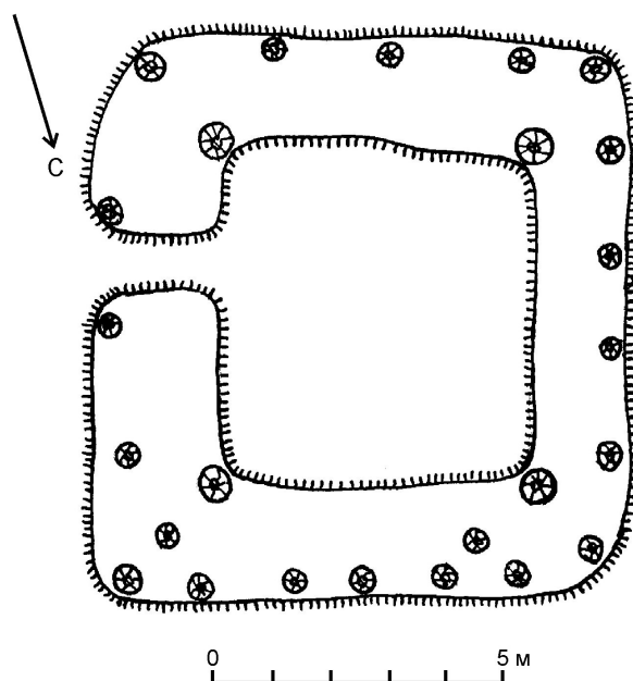
Рис. 3. Жилище № 1 на Волчьем озере [Пытляков, 1955]
